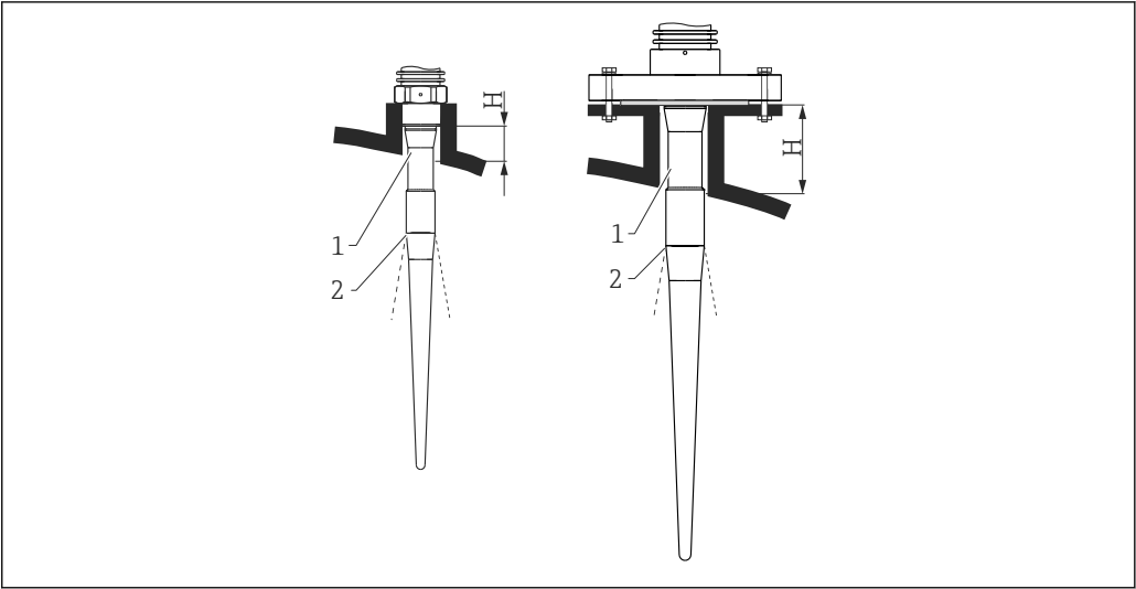
图 17 杆式天线的安装短管长度和管径示意图 (FMR53)
