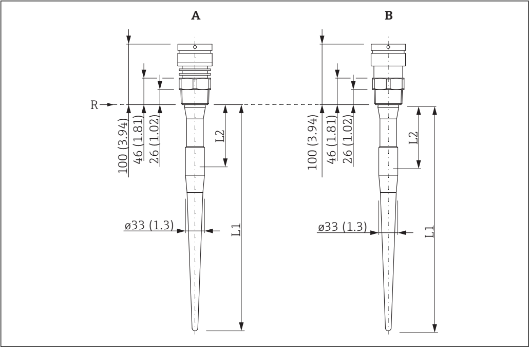
28 带螺纹连接的 FMR53 的外形尺寸示意图；单位：mm (in)
