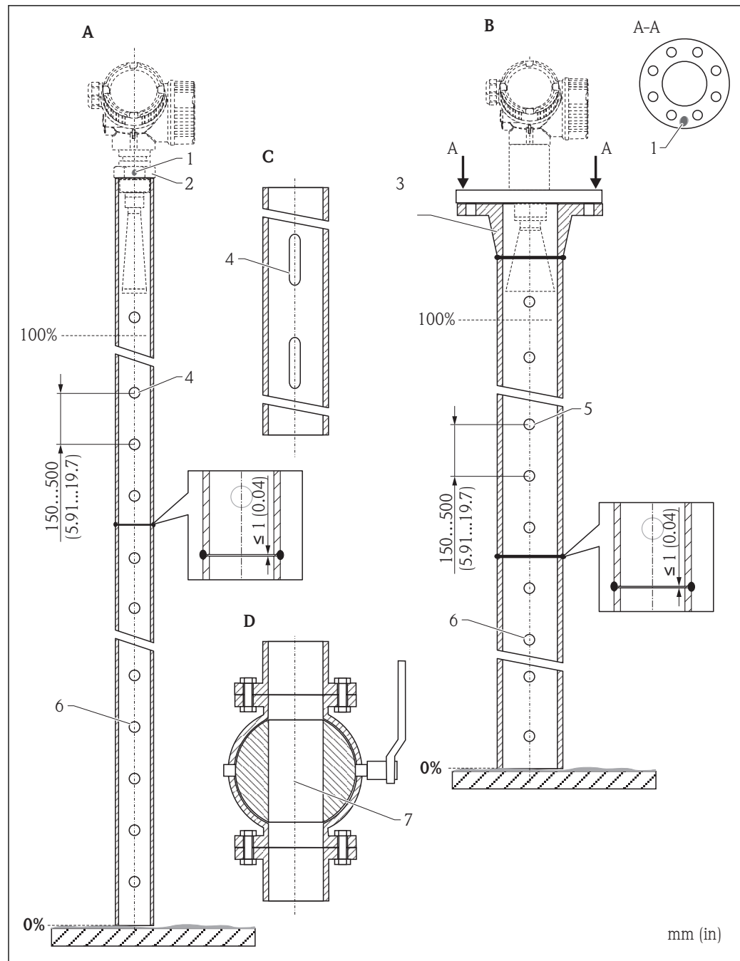
导波管的结构示例
