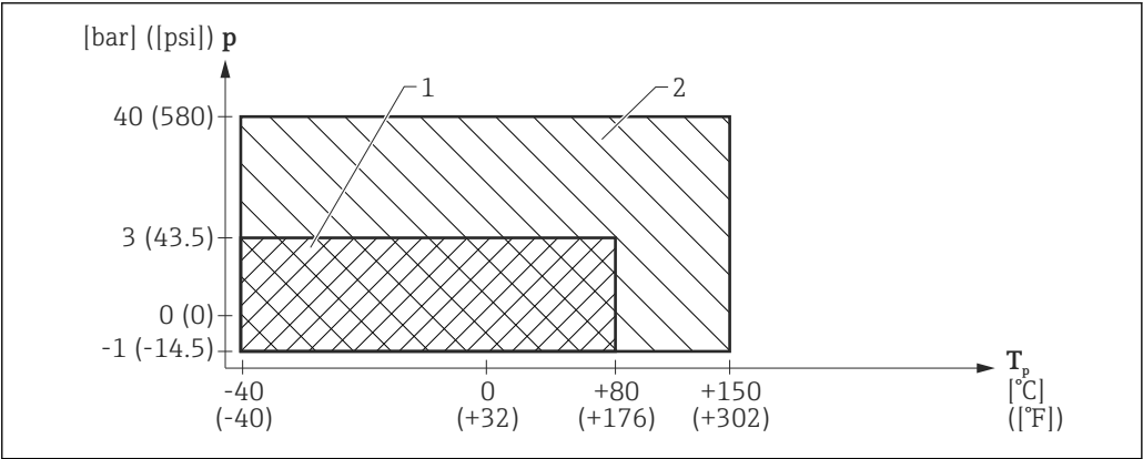
21 FMR53: 允许过程温度和过程压力范围
