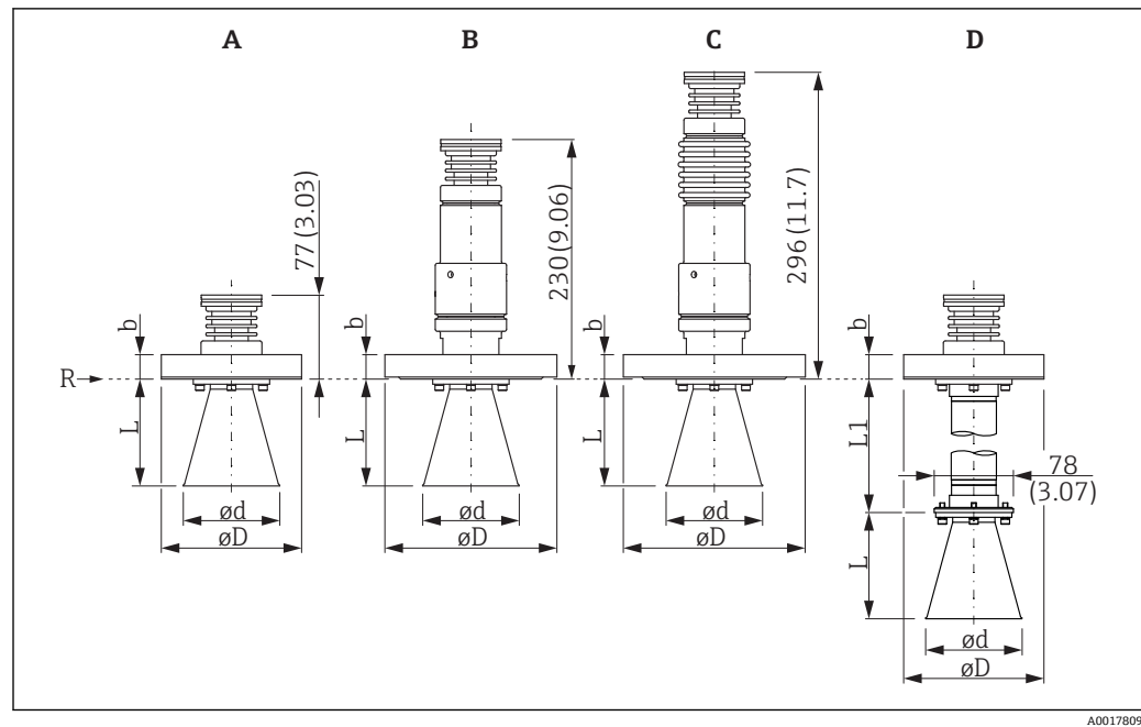
图 29 带螺纹连接的 FMR54 的外形尺寸示意图；单位：mm (in)
