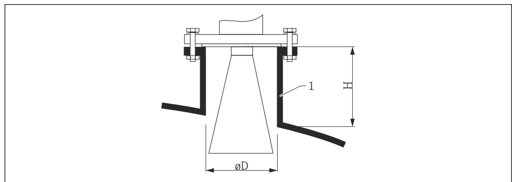
图 18 喇叭天线的安装短管长度和管径 (FMR54) 示意图
