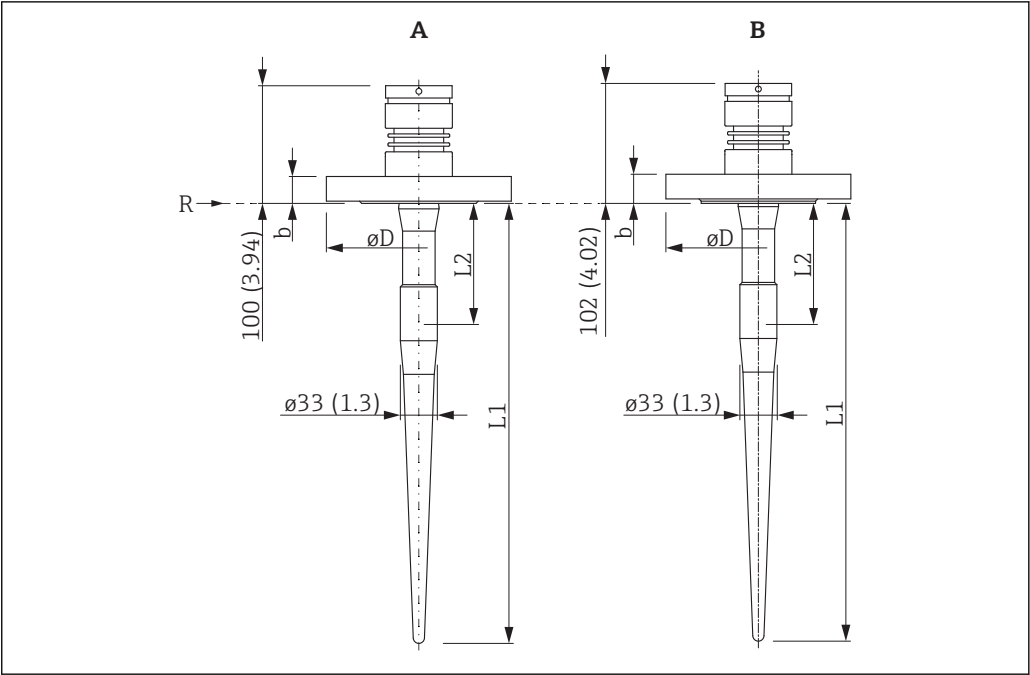
图 27 带螺纹连接的 FMR53 的外形尺寸示意图；单位：mm (in)
