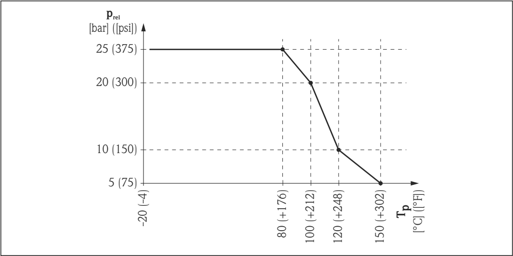
图 23 带平面天线的 FMR54: 允许过程温度和过程压力范围
