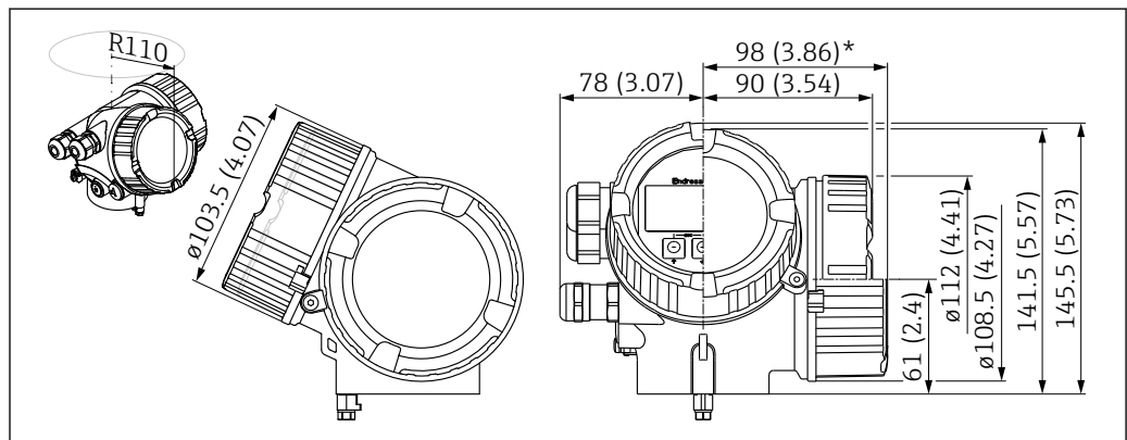
图 26 GT20 外壳 (铝, 带涂层) ; 单位: mm (in)
