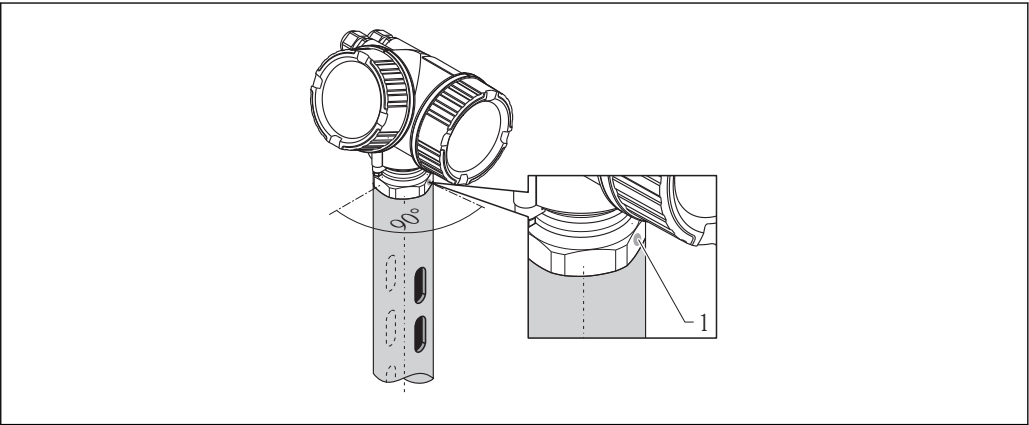
图 19 在导波管中安装
