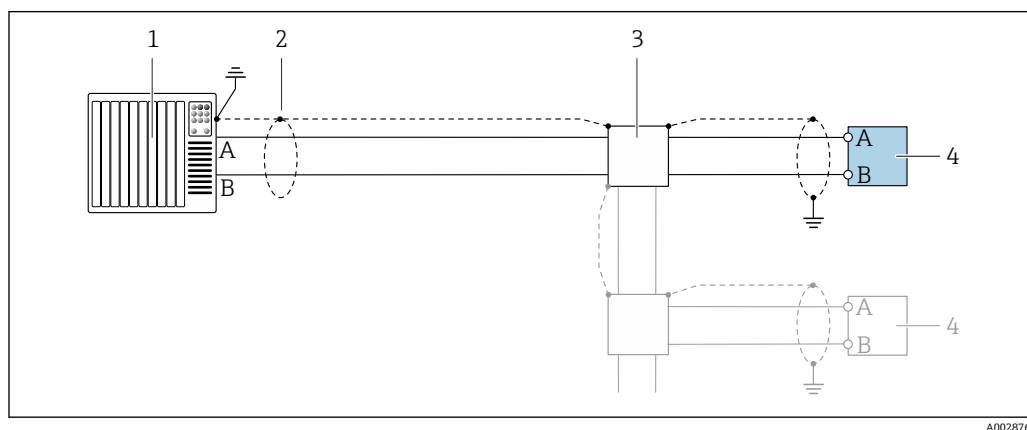
■ 10 Modbus RS485 的连接实例, 在非危险区和 Zone 2; Cl. I, Div. 2 防爆场合中
