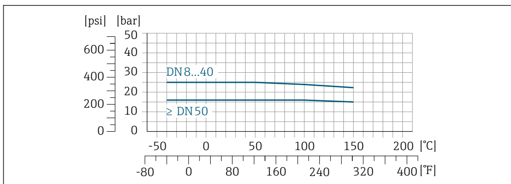
图 27 法兰材质: 1.4404 (316/316L)
