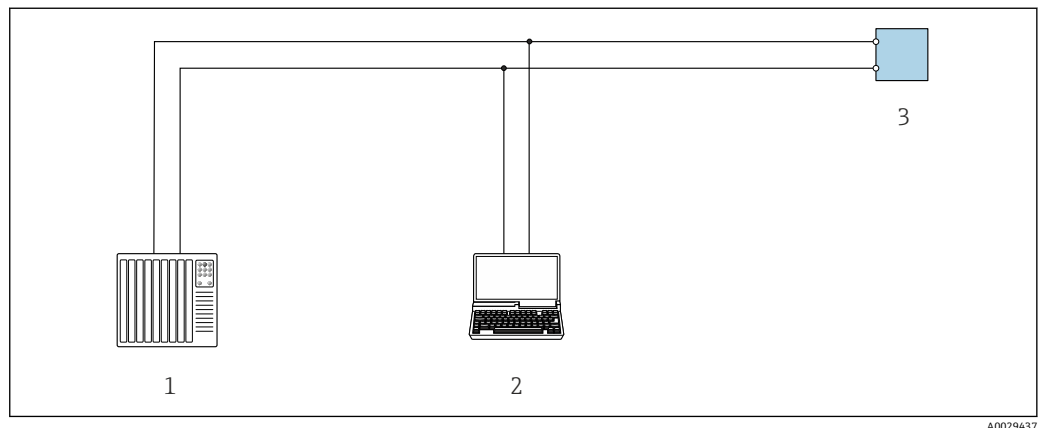
图 52 通过 Modbus-RS485 通信进行远程操作(有源信号)
