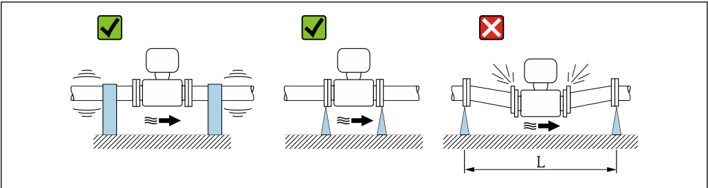
34 避免仪表振动的措施(L > 10 m (33 ft))
