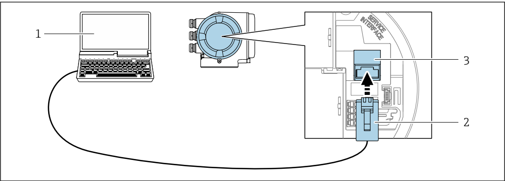
图 53 通过服务接口(CDI-RJ45)操作
