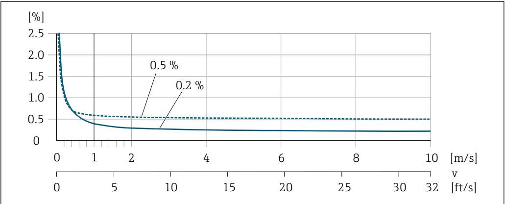
17 最大测量误差(% o.r.)
