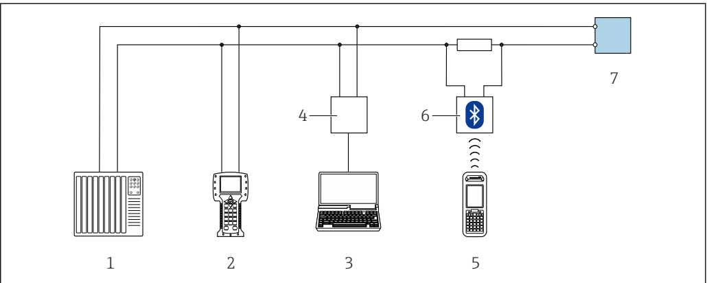
48 通过 HART 通信进行远程操作(有源信号)
