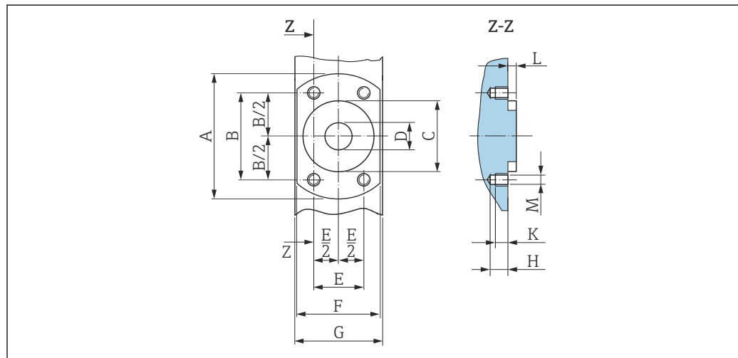
图 40 正视图，无过程连接
