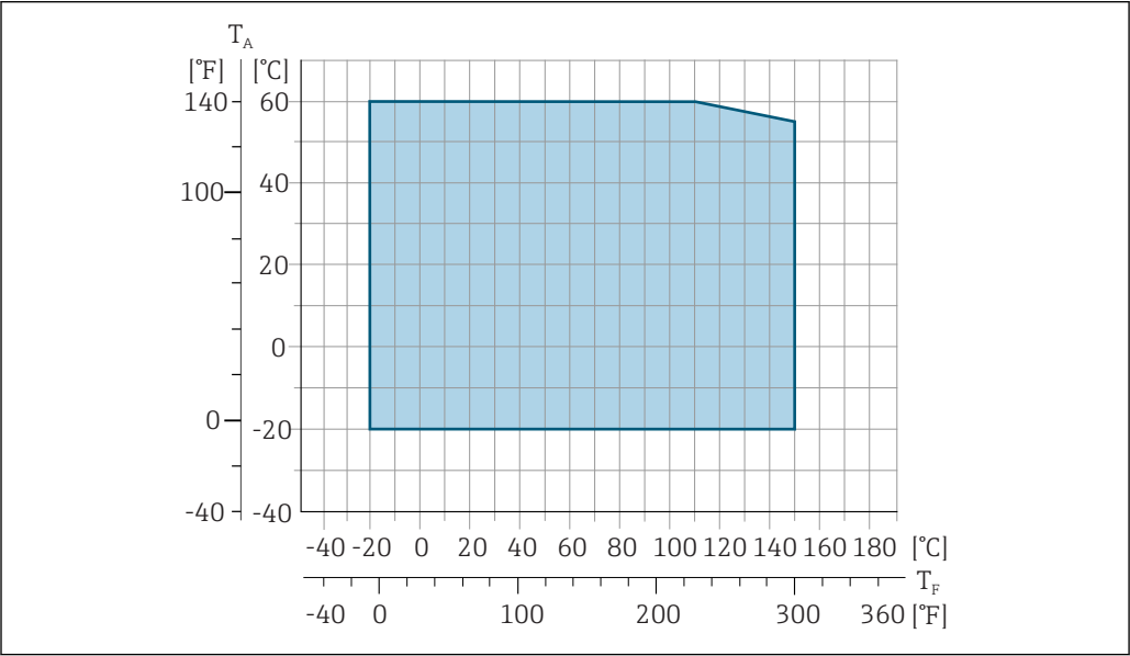
T A 环境温度范围 T F 流体温度
