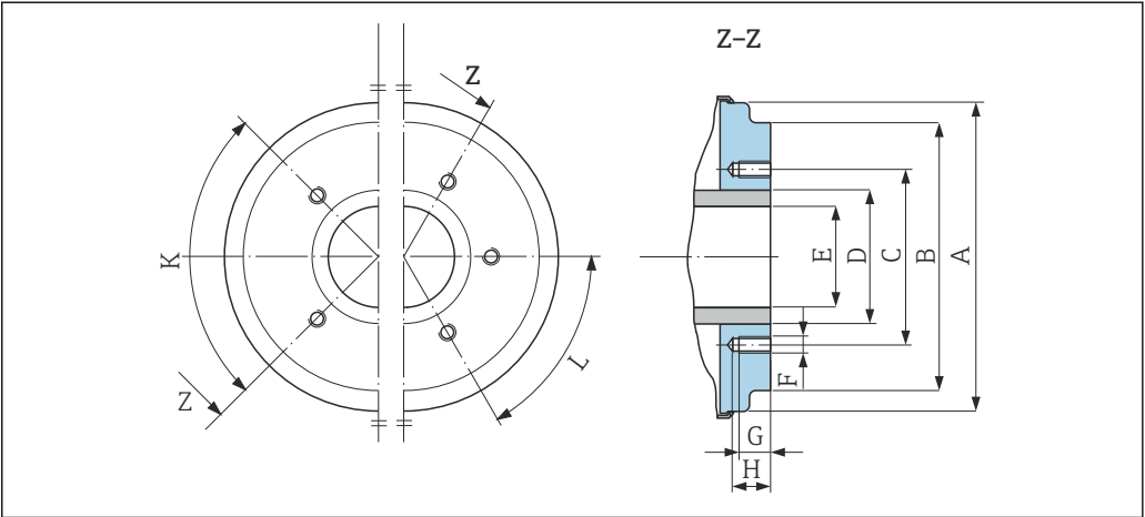
41 正视图，未安装过程连接
