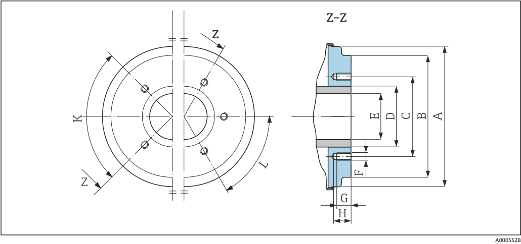
图 36 正视图，未安装过程连接
