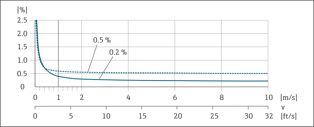
图 21 最大测量误差(% o.r.)
