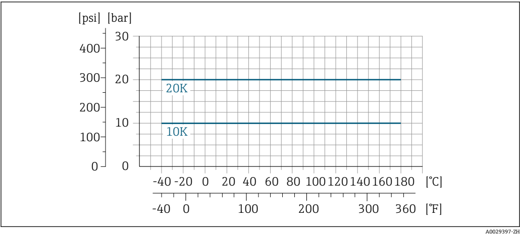
图 36 过程连接材料: 不锈钢 1.0425 (F316L)、碳钢 S235JRG2/HII
