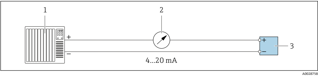
图 8 4...20 mA 有源电流输出的连接实例
