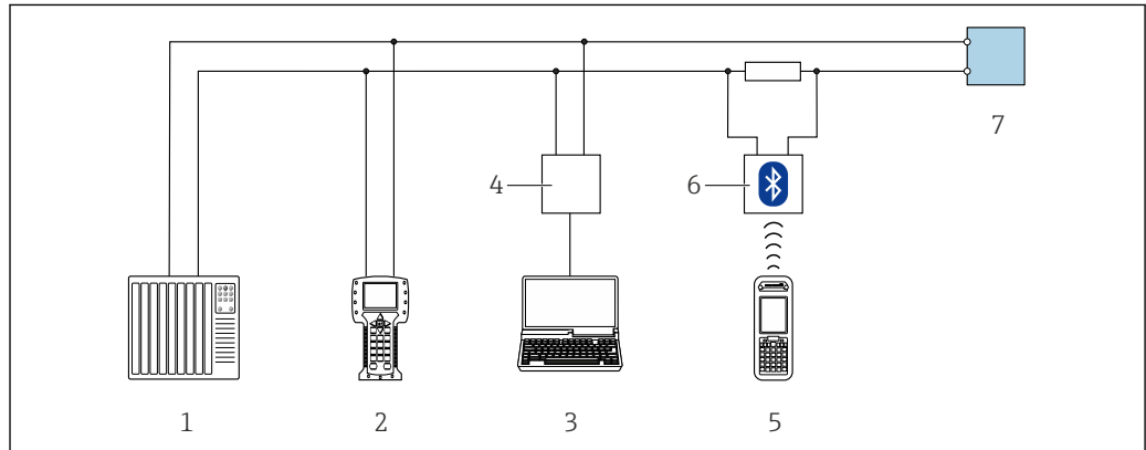
图 43 通过 HART 通信进行远程操作(有源信号)
