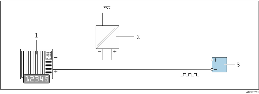
图 10 脉冲/频率输出(无源信号)的连接实例
