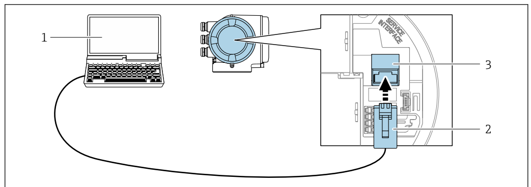
图 49 通过服务接口 (CDI-RJ45) 操作
