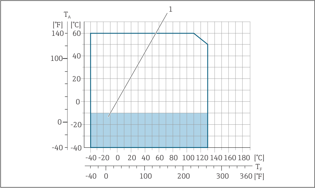
31 PTFE T_A 环境温度范围 T_F 流体温度 1 灰色区域: -10...-40 °C (+14...-40 °F)环境温度范围仅适用于不锈钢法兰
