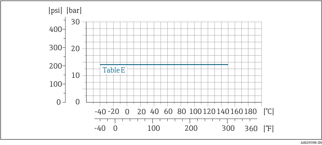
图 37 过程连接材料: 碳钢 A105/S235JRG2/S275JR
