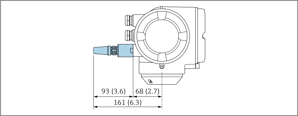
图 40 单位: mm (in)
