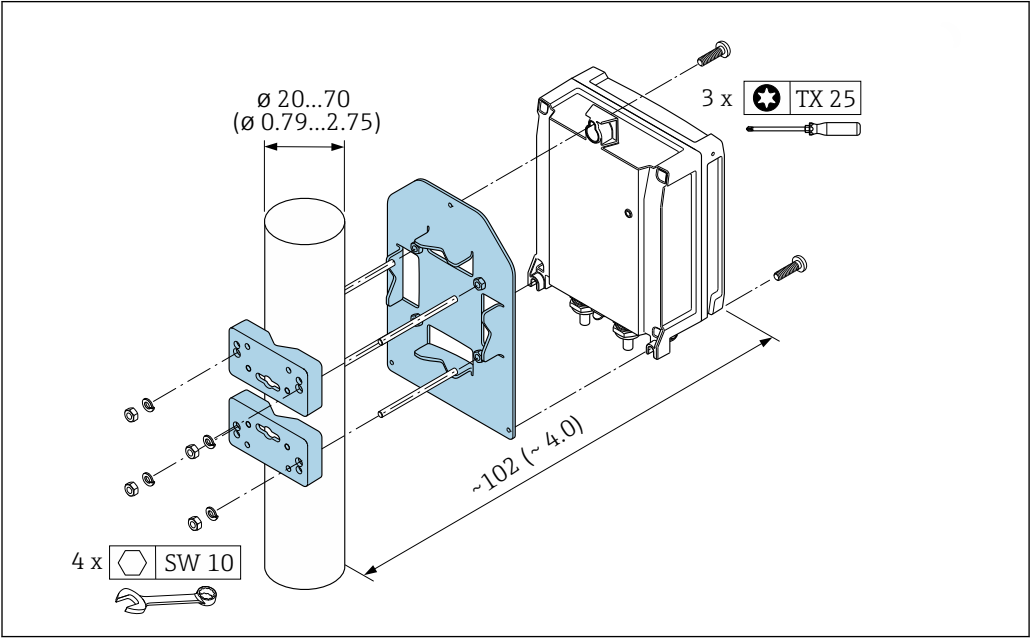
图 24 单位: mm (in)
