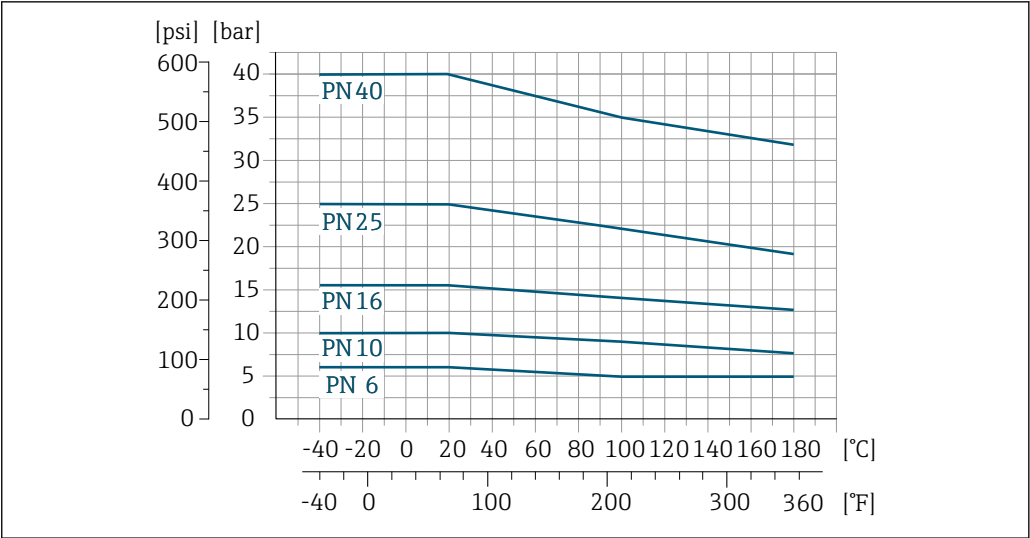
33 过程连接材料: 不锈钢 1.4571 (F316L)
