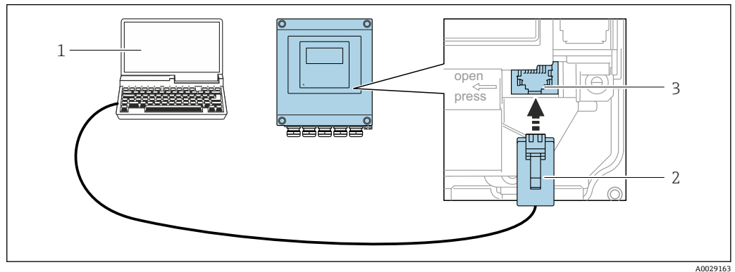
图 48 通过服务接口 (CDI-RJ45) 操作
