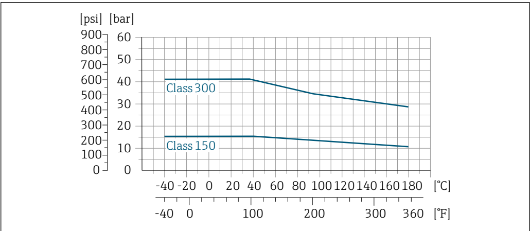
35 过程连接材料: 不锈钢 F316L
