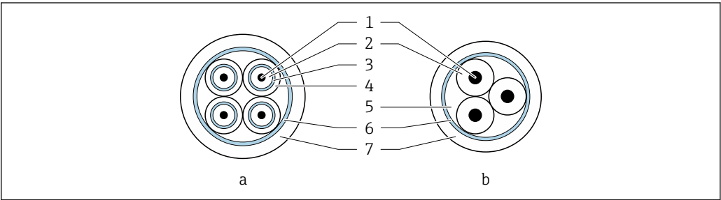
图 20 电缆横截面积
