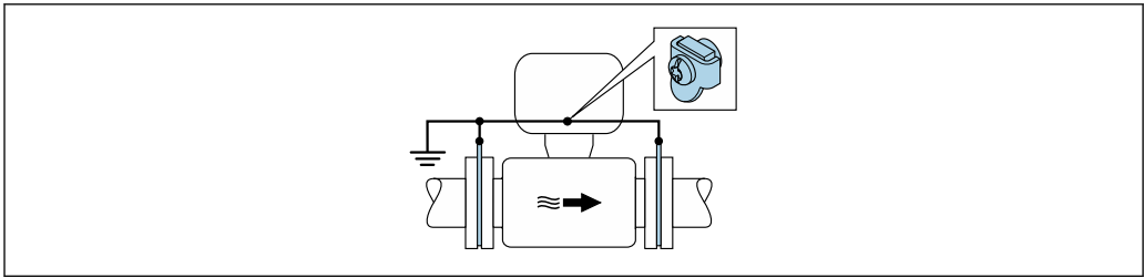
图 19 通过接地端子和接地环实现系统电势平衡
