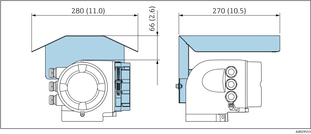
图 29 Proline 500 的防护罩
