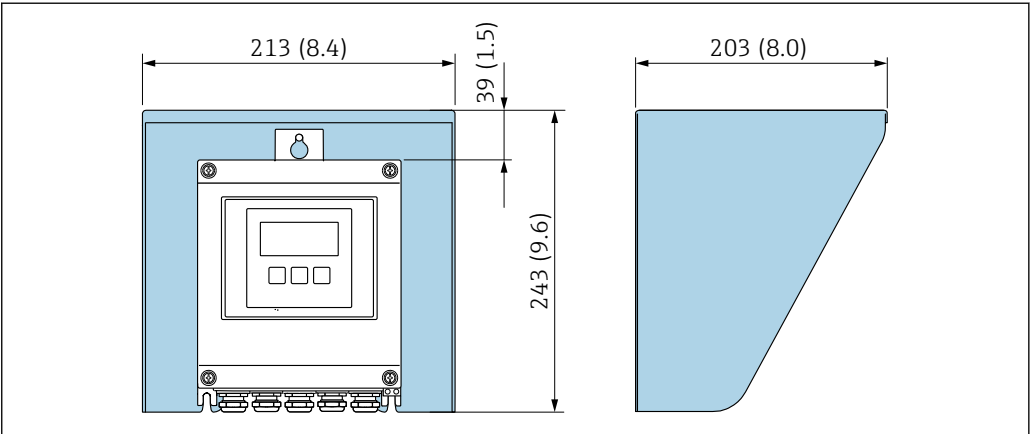
28 Proline 500 (数字式)的防护罩
