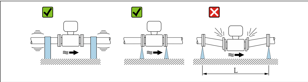
图 38 避免仪表振动的措施(L > 10 m (33 ft))
