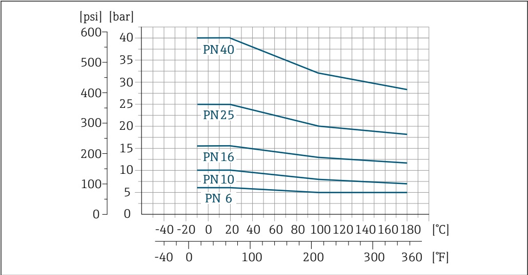
32 过程连接材料: 碳钢 FE410WB/S235JRG2、Alloy C22 合金 2.4602 (UNS N06022)
